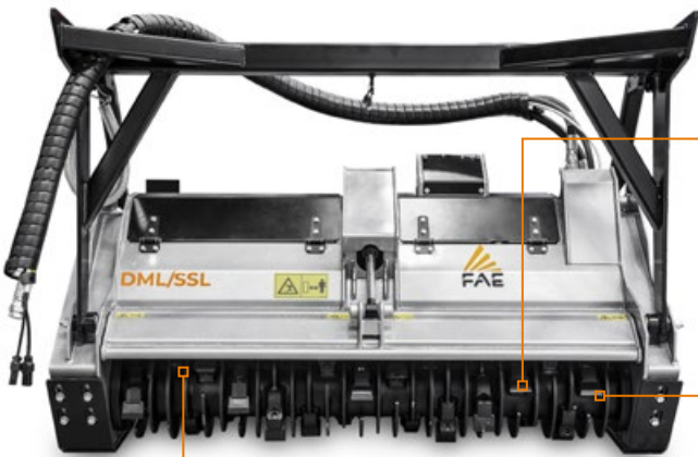
Rotor avec technologie Bite Limiter productivité maximale et demande de puissance minimale grâce aux inserts spéciaux en acier haute résistance et aux lames de type BL/MINI (DML/SSL/BL et DML/SSL/BL/SONIC)
